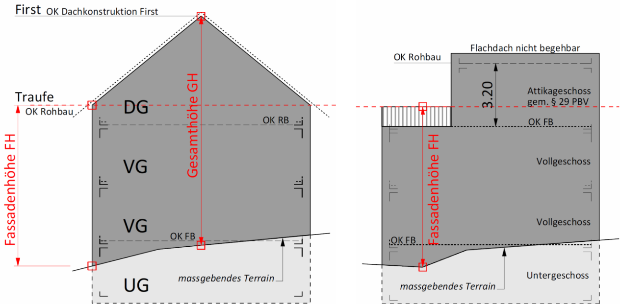
Schrägdach
